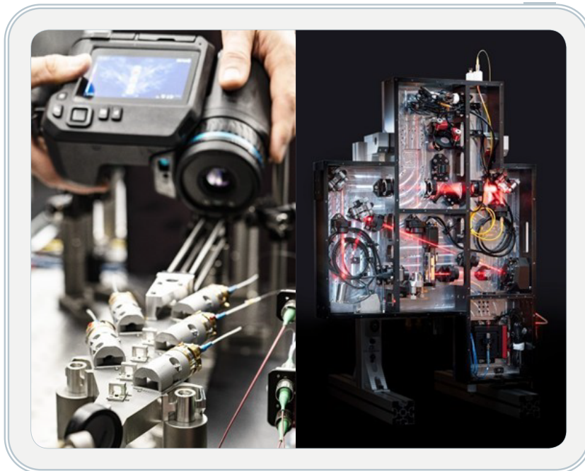
그림 7. (좌) 프라운호퍼(Fraunhofer)IOF에서 개발한 파장 다중화기(WDM)는 위성 간 통신을 향후 더 먼 거리에 걸쳐 더 높은 데이터 전송률을 실현할 수 있게 함. (우) 보정 광학 모듈(adaptive optical module). 위성상과 기지국 사이의 데이터 통신시 자유 공간 전송 중 대기 난류로 인해 교란된 파면을 보정함
