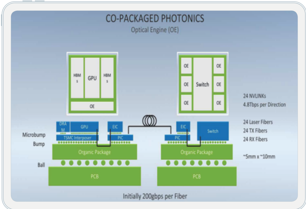
그림 6. 코패키징 포토닉스는 광학엔진(Optical Engine, OE)을 반도체와 같은 다른 부품들과 함께 하나의 패키지에 통합하는 기술임. 이를 통해 전자신호 대신 빛을 이용하여 데이터를 더 빠르고 효율적으로 전송할 수 있음 14)
