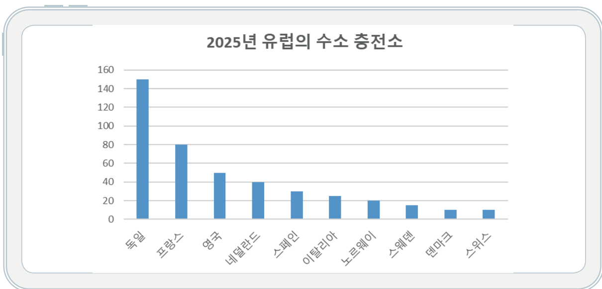
그림 7. 유럽의 국가별 수소충전 인프라(2025년) 14)
