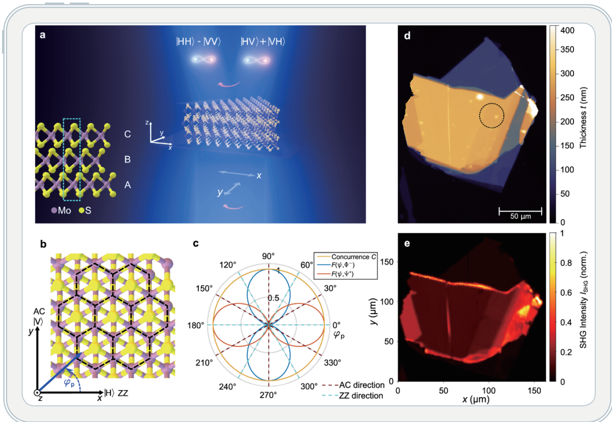
그림 9. 튜닝 가능한 전이 금속 칼코겐화합물 얹힌 광자 쌍 광원(A tunable transition metal dichalcogenide entangled photon-pair source) 16) 은 2차원 물질인 전이 금속 칼코겐화합물(TMD)을 사용하여 얹힌 광자 쌍을 생성하는 혁신적인 접근 방식을 제시함. 연구진은 TMD의 고유한 광학적 특성을 활용하여 기존 방식보다 훨씬 효율적으로 얹힌 광자 쌍을 생성하는 데 성공함. 특히, 생성된 광자 쌍의 파장과 특성을 정밀하게 튜닝할 수 있다는 점은 양자 광학 시스템의 유연성을 크게 향상시키고, 다양한 응용 분야에 적용 가능성을 넓혔음 16)
